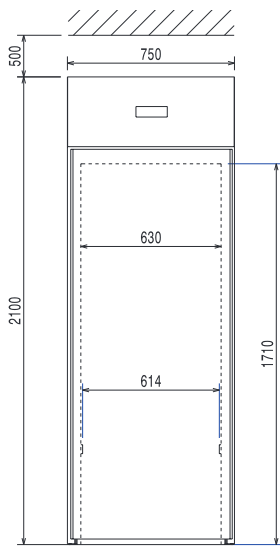
Front aanzicht
